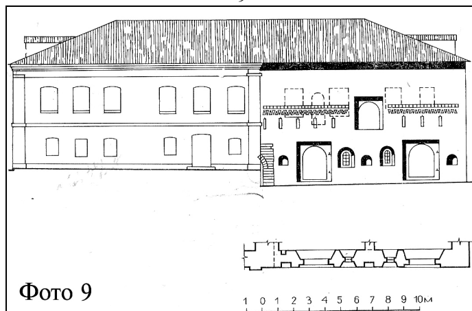
Рис.9. Реконструкция восточного фасада сохранившейся части Погребного корпуса.
