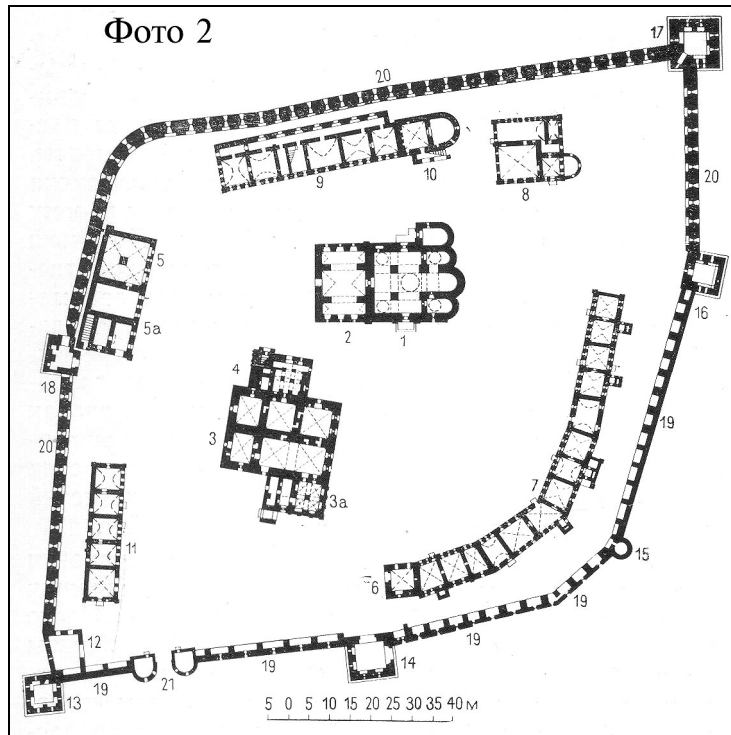
Рис.2. Планировка монастыря. 1 – собор Рождества Богородицы, 1586 г.; 2 – трапезная (паперть) собора, 1837; 3 – трапезная с церковью Рождества Христова, 1511 г.; 3а – паперти трапезной, XVI в.; 4 – колокольня, 1690 г.; 5 – погребной корпус, XVI в.; 5а – перестроенная часть погребного корпуса, XIX в.; 6 – сохранившийся фрагмент разобранной церкви Пафнутия с пристройкой, XVI в.; 7 – юго-восточные братские кельи, XVII в.; 8 – больничные палаты с церковью Ильи, 1670 г.; 9 – настоятельские палаты, XVII в.; 10 – церковь Митрофана, 1760 г.; 11 – западные братские кельи, XVII в.; 12 – поваренная палата, XVII (?) в.; 13 – Поваренная башня, XVI в.; 14 – Георгиевская башня, XVI в.; 15 – Круглая башня, XVI в.; 16 – Оружейная башня, XVI в.; 17 – Сторожевая башня, XVII в.; 18 – Тайницкая башня, XVII в.; 19 – прясла крепостных стен, XVI в.; 20 – прясла крепостных стен, XVII в.; 21 – Проломные («Водяные») ворота, XVII–XIX вв.
