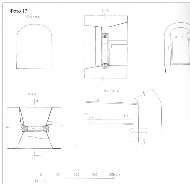
Рис.17. Западные братские кельи XVII в. Обмерный чертеж окна первого этажа в западной стене с первоначальной дубовой колодой.
